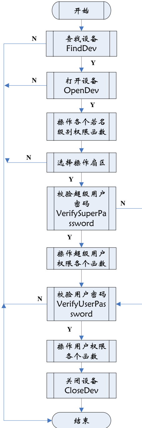
图 3-1 函数调用总体流程图
